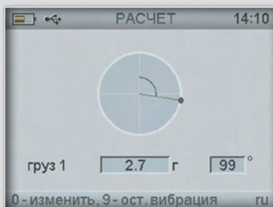
Расчет места установки уравновешивающей массы
