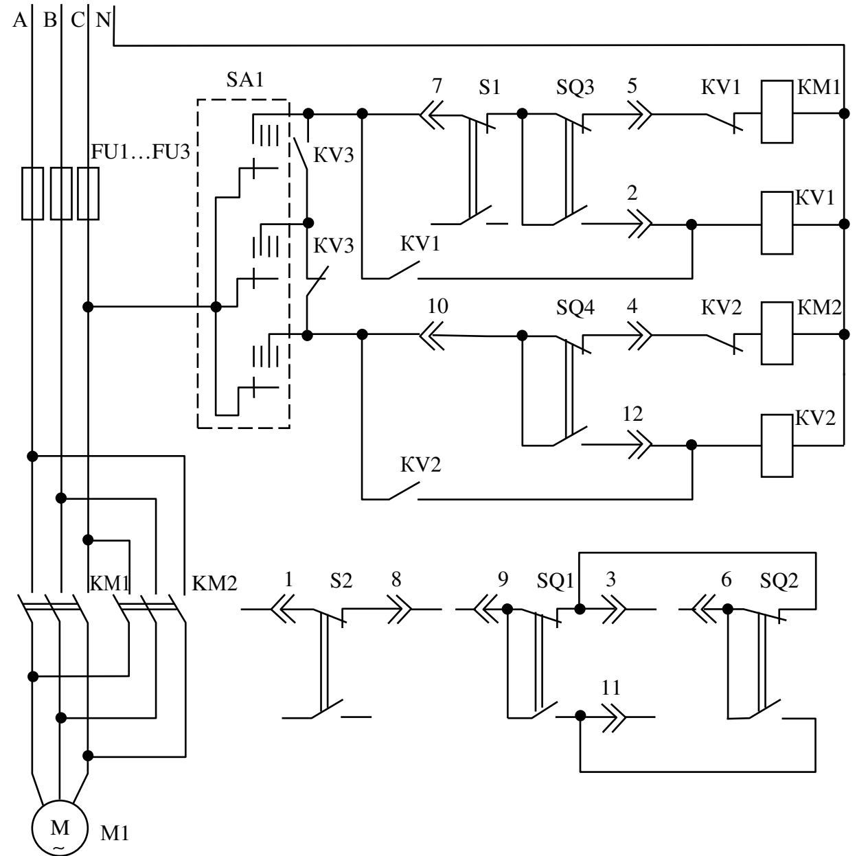
Рисунок 6 — Принципиальная электрическая схема электроприводов
