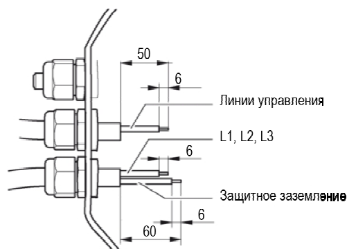
III. 1. Рекомендуемая длина зачистки изоляции в мм (внутри клеммной коробки)
