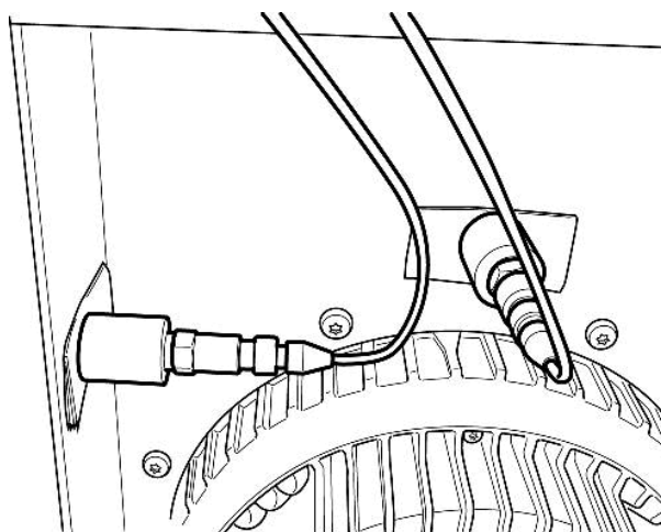
Иллюстрация 4: Примерное представление измерения параметров вибрации. Расположение датчиков зависит от соответствующего устройства и монтажного положения.
