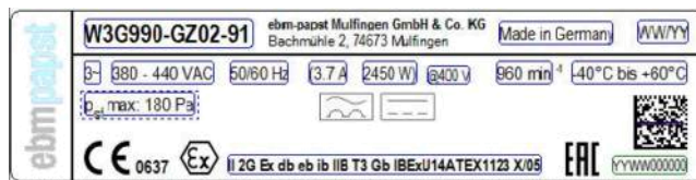
Иллюстрация 1: Характеристики на заводской табличке
