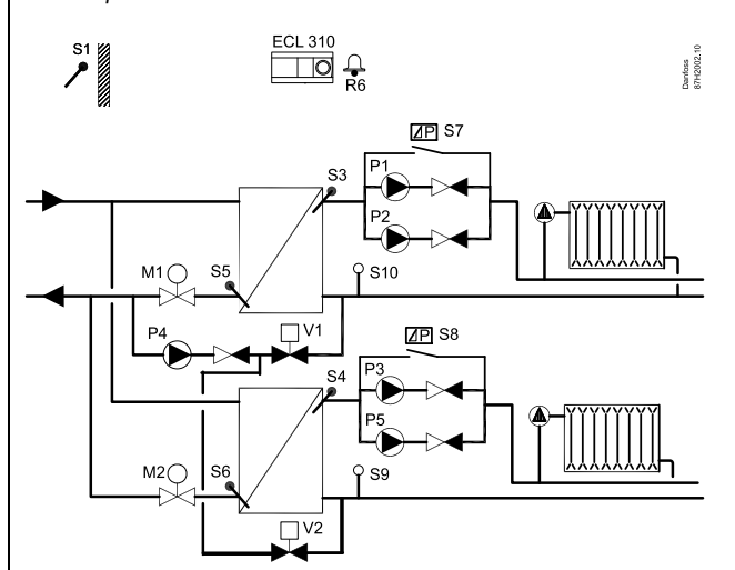
Стандартная схема A361.1
