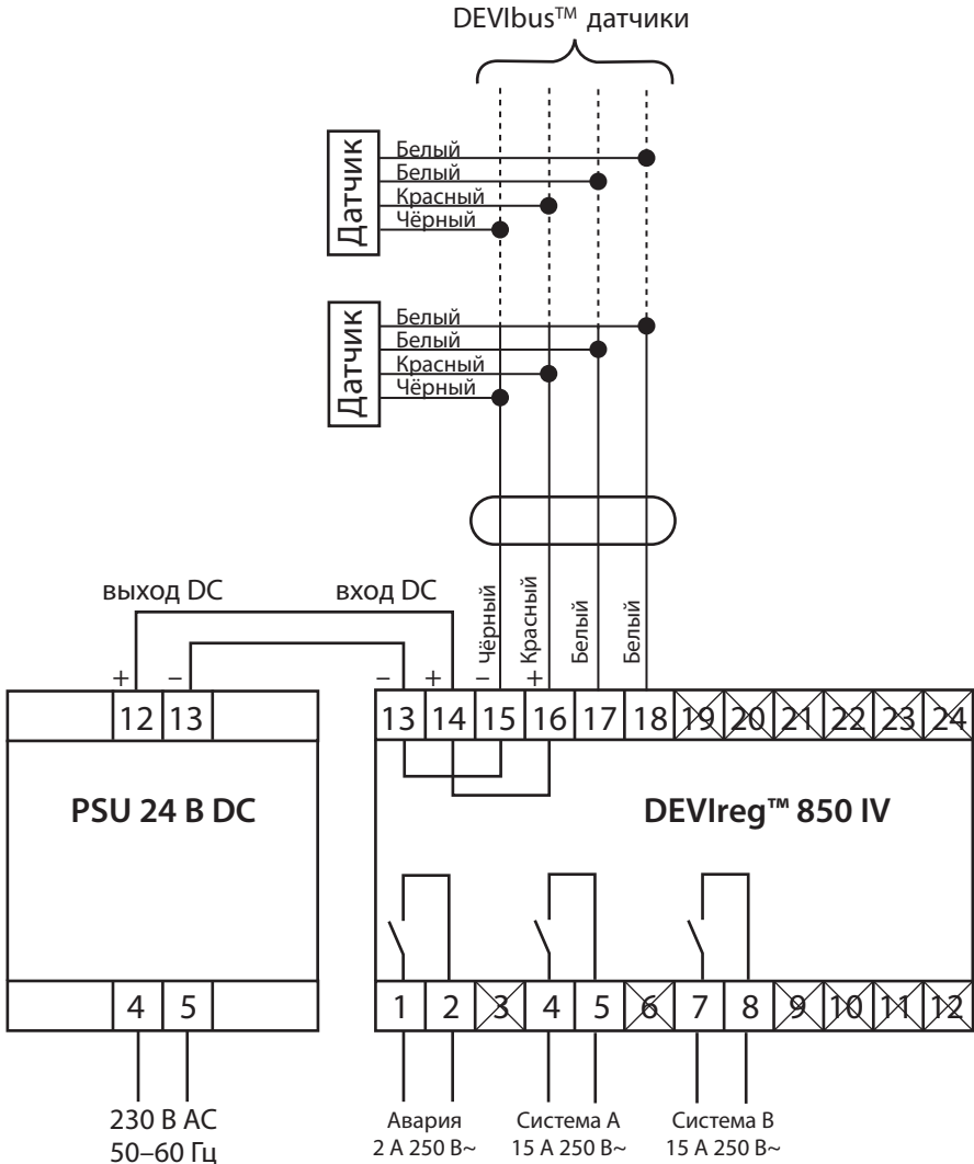
Рис. А - Схема соединений DEVIreg™ 850
