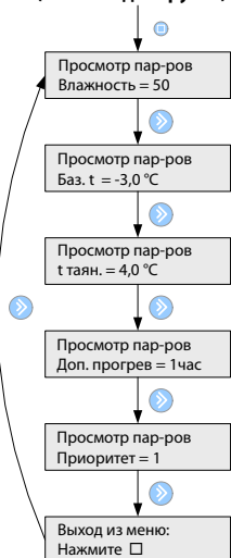
Просмотр параметров системы (Система для грунта)
