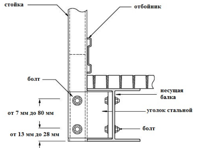
Крепление на двутавровую балку посредством стального уголка
