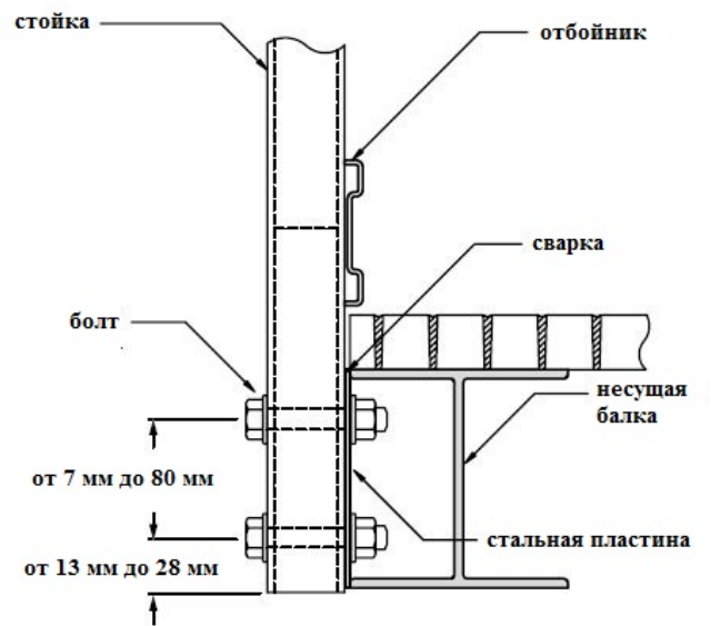
Крепление на двутавровую балку с помощью приваренной стальной пластины
