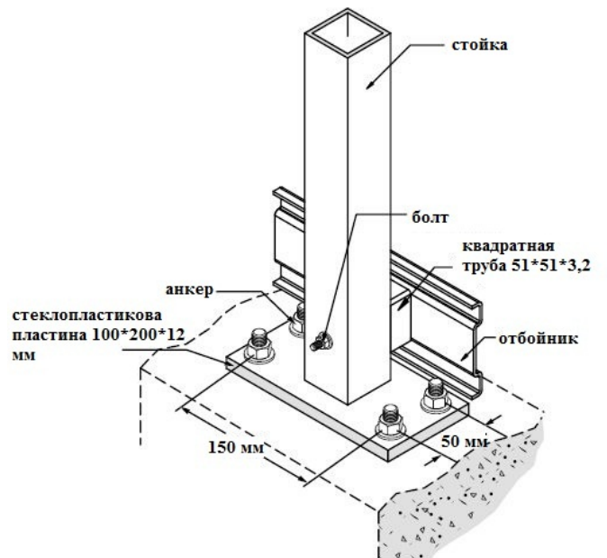
Крепление с помощью стеклопластиковой пластины
