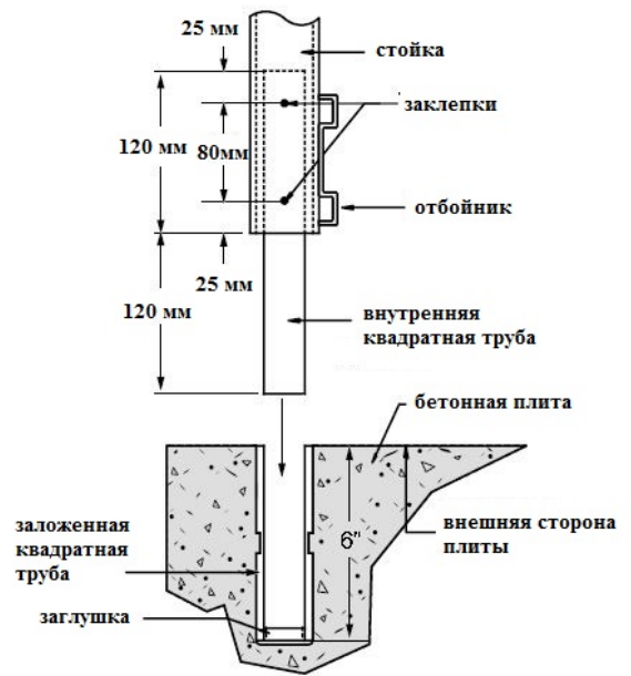
Крепление на бетонное основание с помощью квадратной трубки и заглушки
