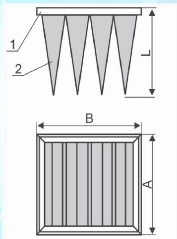
Рис.2 Схема фильтра ФЯК-СП.
