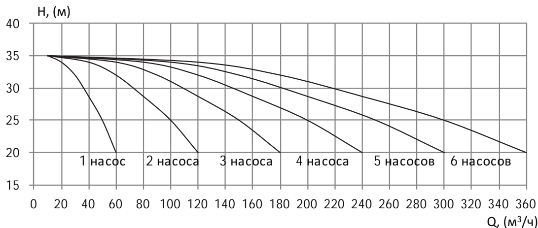
УНВ МНС 65–50/160 5,5 кВт
