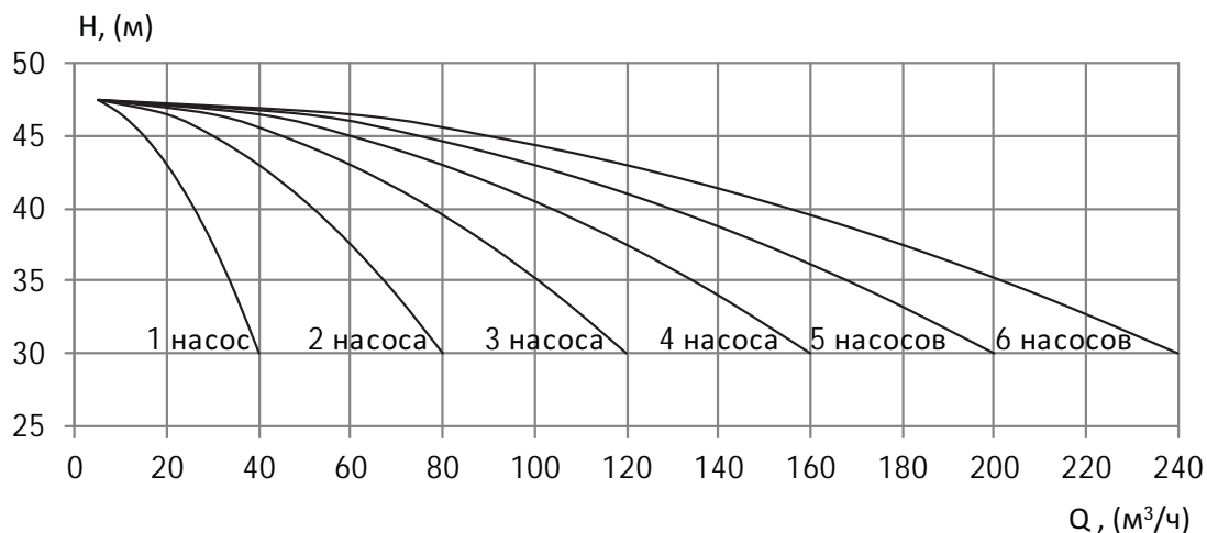
УНВ МНС 65–40/200 7,5 кВт
