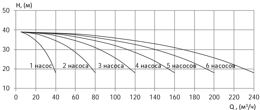
УНВ МНС 65–40/160 4,0 кВт
