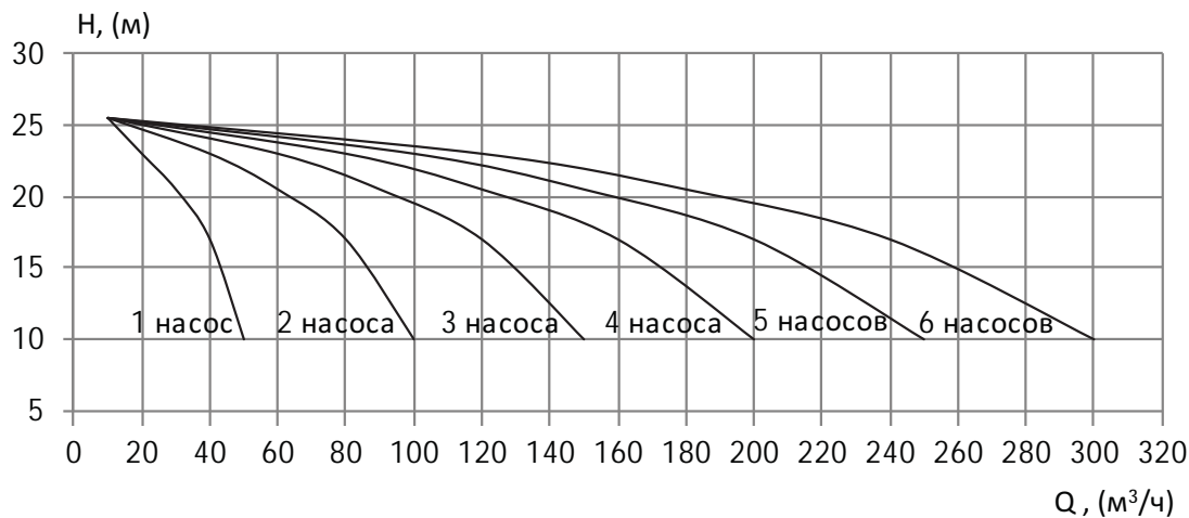
УНВ МНС 65–50/125 3,0 кВт
