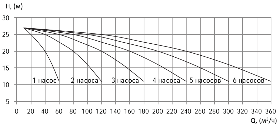
УНВ МНС 65–50/125 4,0 кВт
