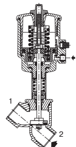
Функция NЗ, вход под диском, приводы 63, 90 и 125 мм
