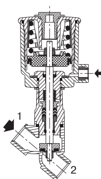
привод 50 мм
