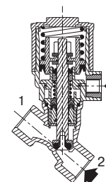
Функция NЗ, вход под диском, приводы 32, 50 мм
