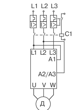
Главный пуск и останов выбегом
