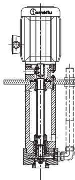
Модель VCP-M в разрезе
