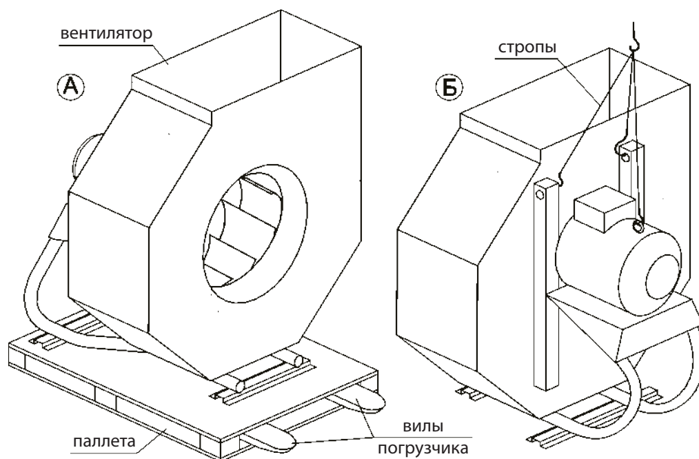
Рисунок 1. Погрузка(выгрузка) вентилятора: А - виловым погрузочным приспособлением; Б - краном.
