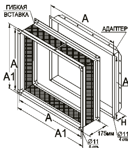
Рисунок 6. Вставка гибкая квадратная с адаптером
