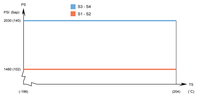
АХР14 – график давления/температуры, сертификация UL
