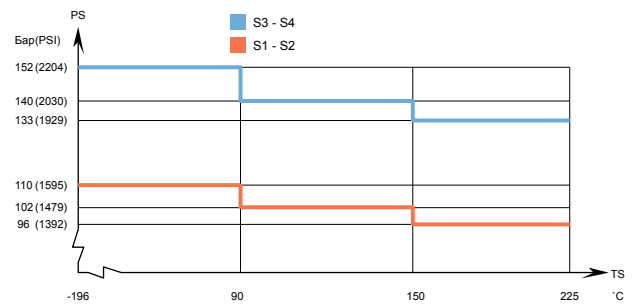
АХР14 – график давления/температуры, сертификация PED (90 и 150)
