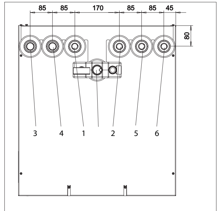
Подключение гидро модуля (вид сверху)
