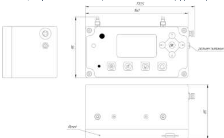
Рисунок 1. Габаритный чертеж
