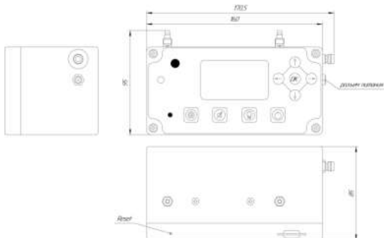
Рисунок 1. Габаритный чертеж
