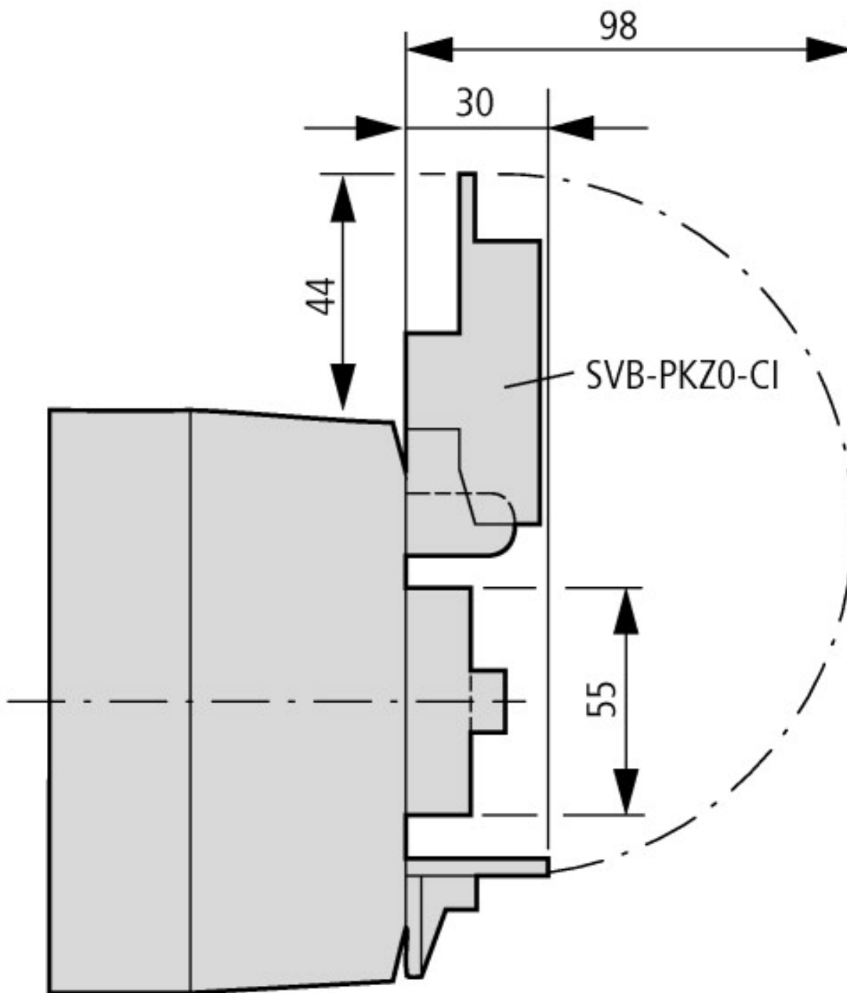
Изолированный корпус для монтажа на поверхность
