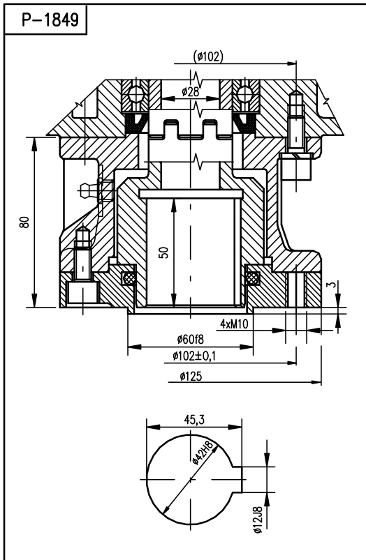
F10 - вид B1; ISO 5210
