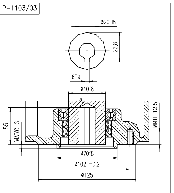
F10 – вид E; ISO 5210
