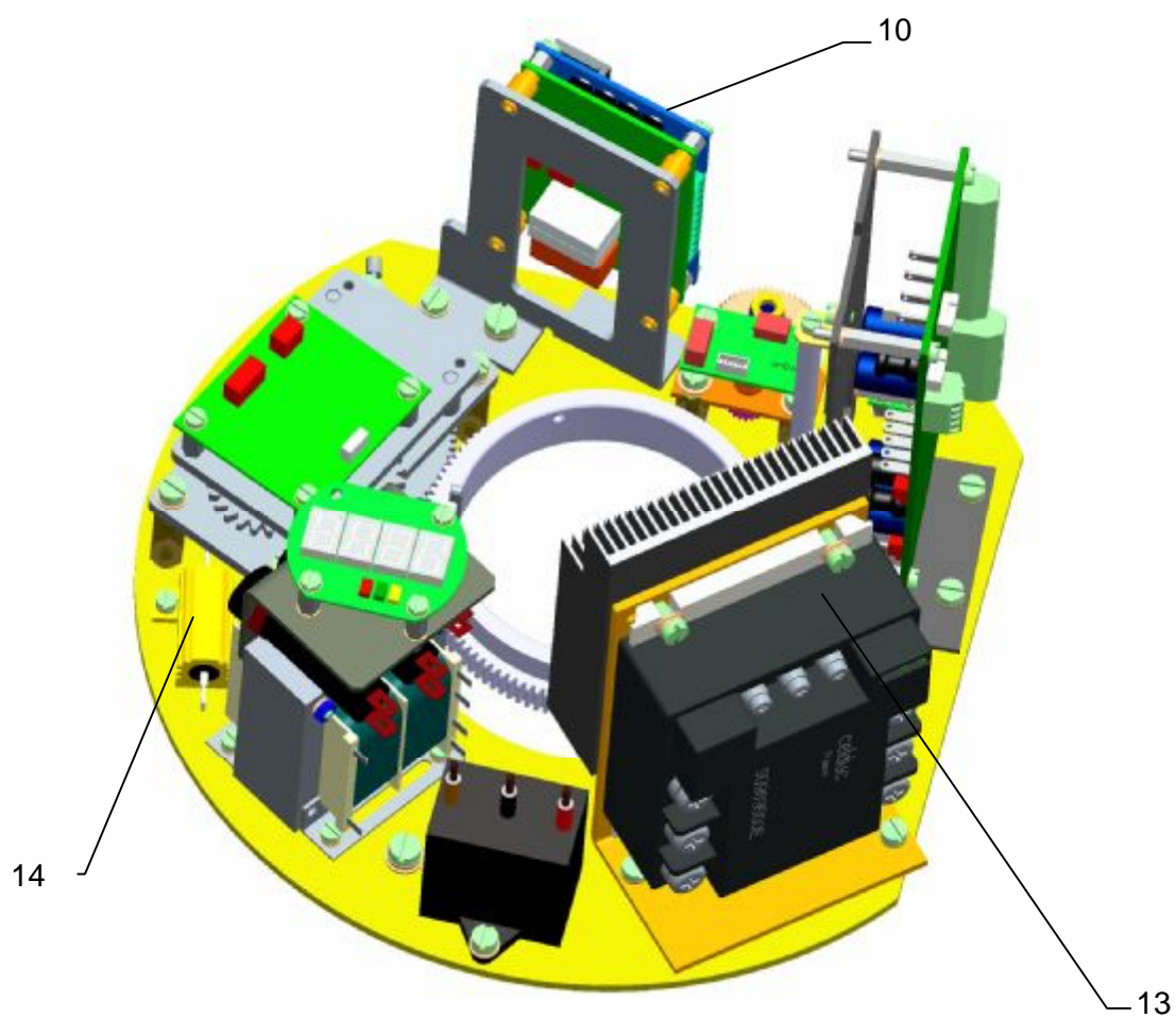
Рис.3а - MOR 5PA-Ex
