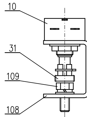
Рис. 7 – Узел датчика
