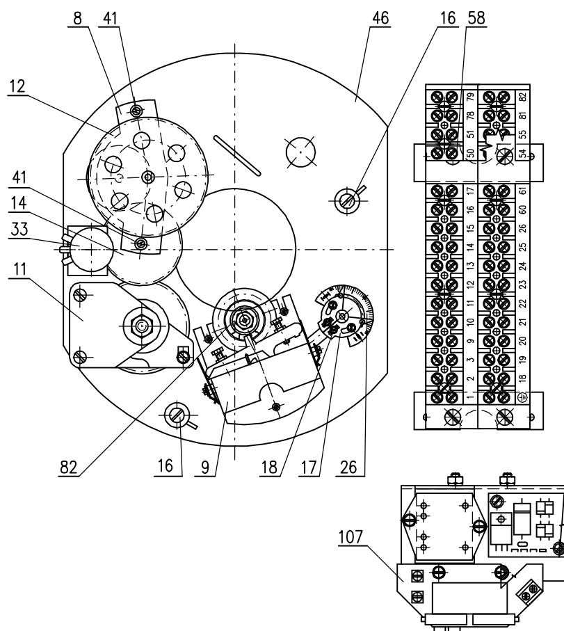
Рис. 3 – Панель управления
