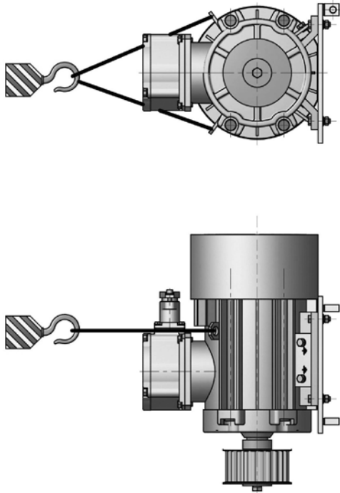
Схема строповки электродвигателя с плиты опорной
