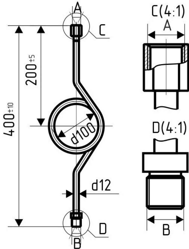
Отвод \text{O}\phi 100\text{B}-1
