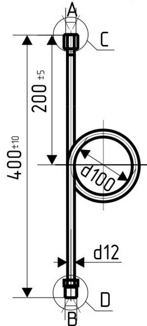
Отвод \text{O}\phi 100\text{B}-2
