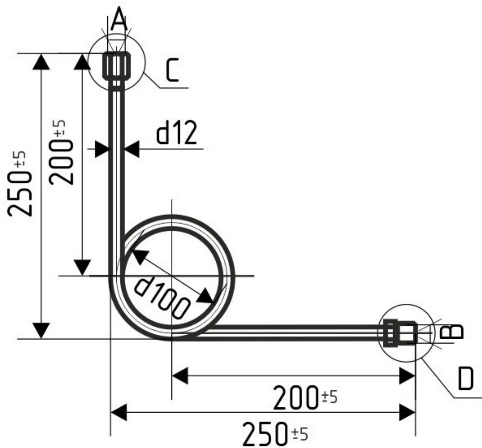
Отвод \text{O}\phi 100\text{B}-3
