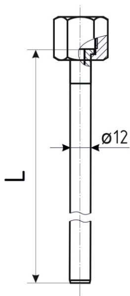
вариант «под приварку»
