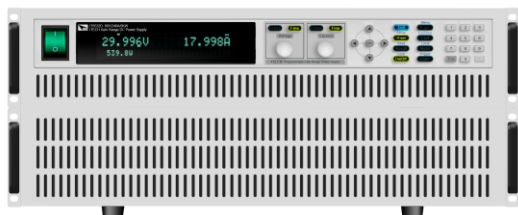
АКИП-1149-750-30
