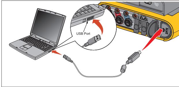
Рисунке 8. Подключение Power Logger к ПК
