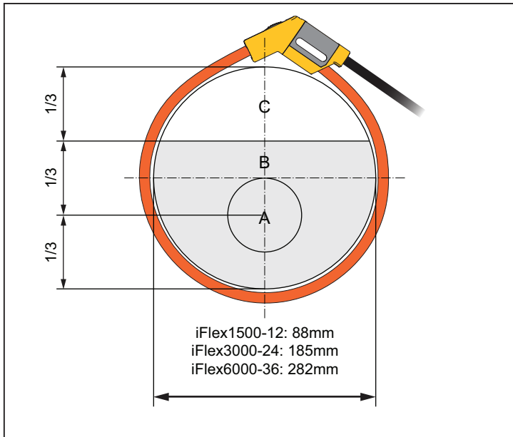
Рисунке 9. Просвет датчика iFlex
