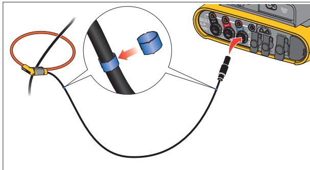
Рисунке 4. Измерительные провода с цветовой кодировкой
