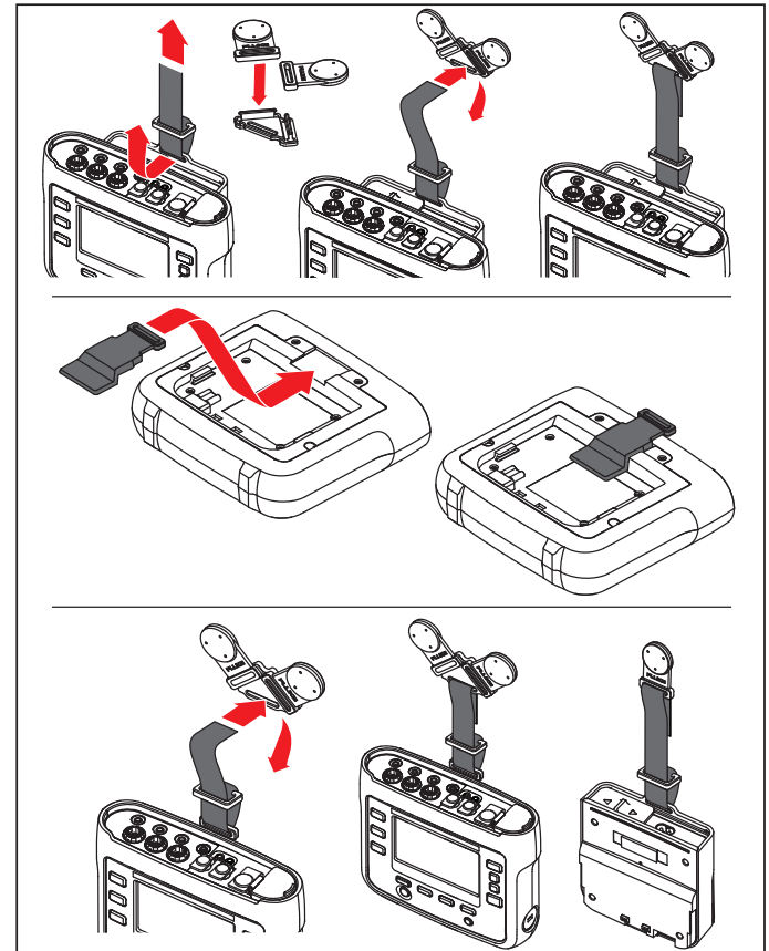
Рисунке 2. Комплект магнитной подвески
