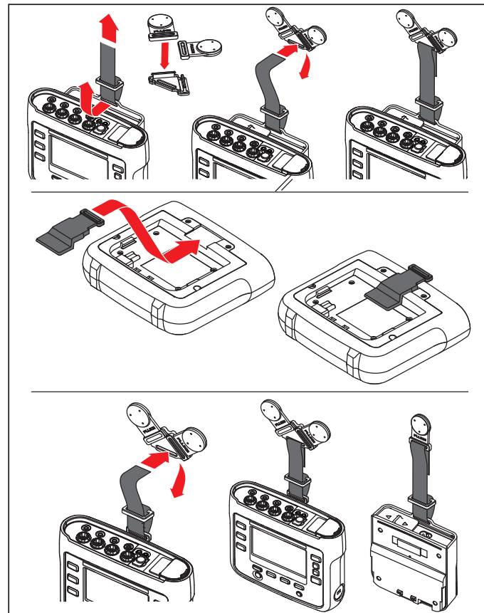
Рисунок 2. Комплект магнитной подвески
