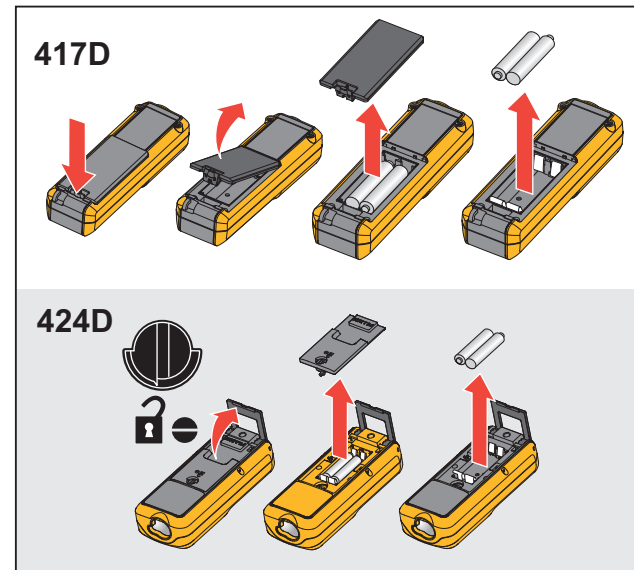
Рисунок 15. Замена батарей
