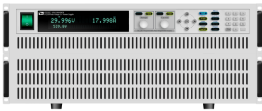
АКИП-1149А-80-240
