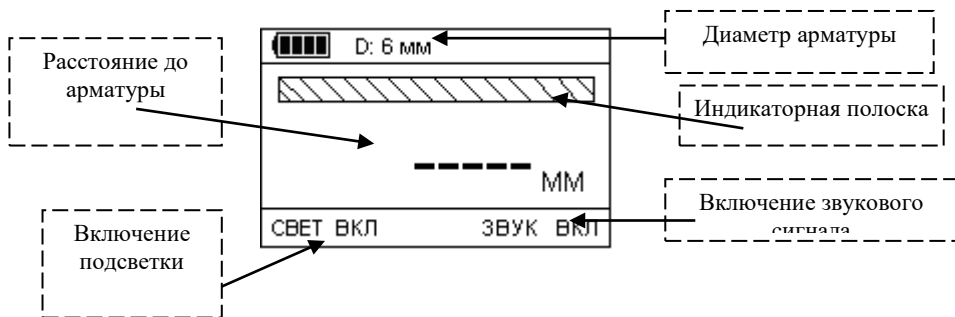
Рисунок 2.8 – Режим сканирования
