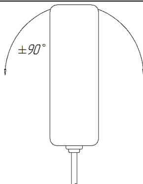
Рисунок 2.6 – Поворот преобразователя при сканировании объекта контроля
