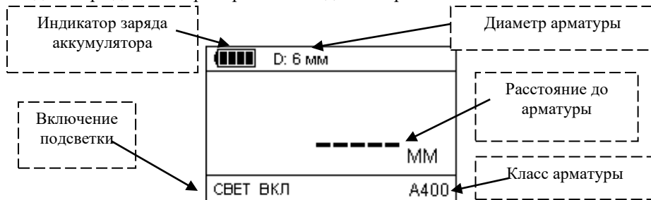
Рисунок 2.4 – Режим измерения глубины залегания арматуры при известном ее диаметре
