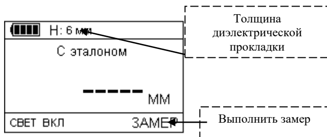
Рисунок 3.2 – Выполнение замера через эталонный образец
