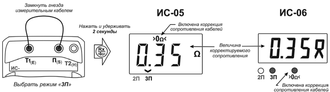
Рисунок 3 – Коррекция сопротивления измерительного кабеля (3П)
