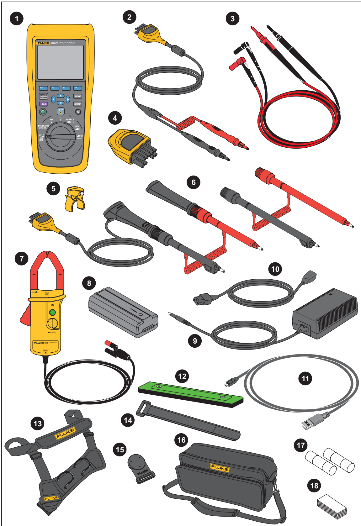
Рис. 1-1. Стандартное оборудование
