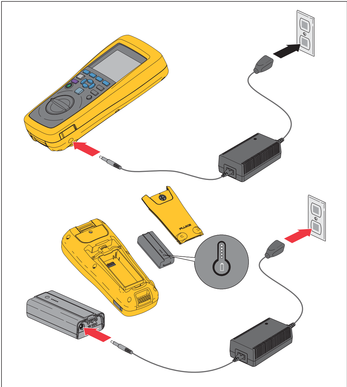
Рис. 7-3. Зарядка батареи
