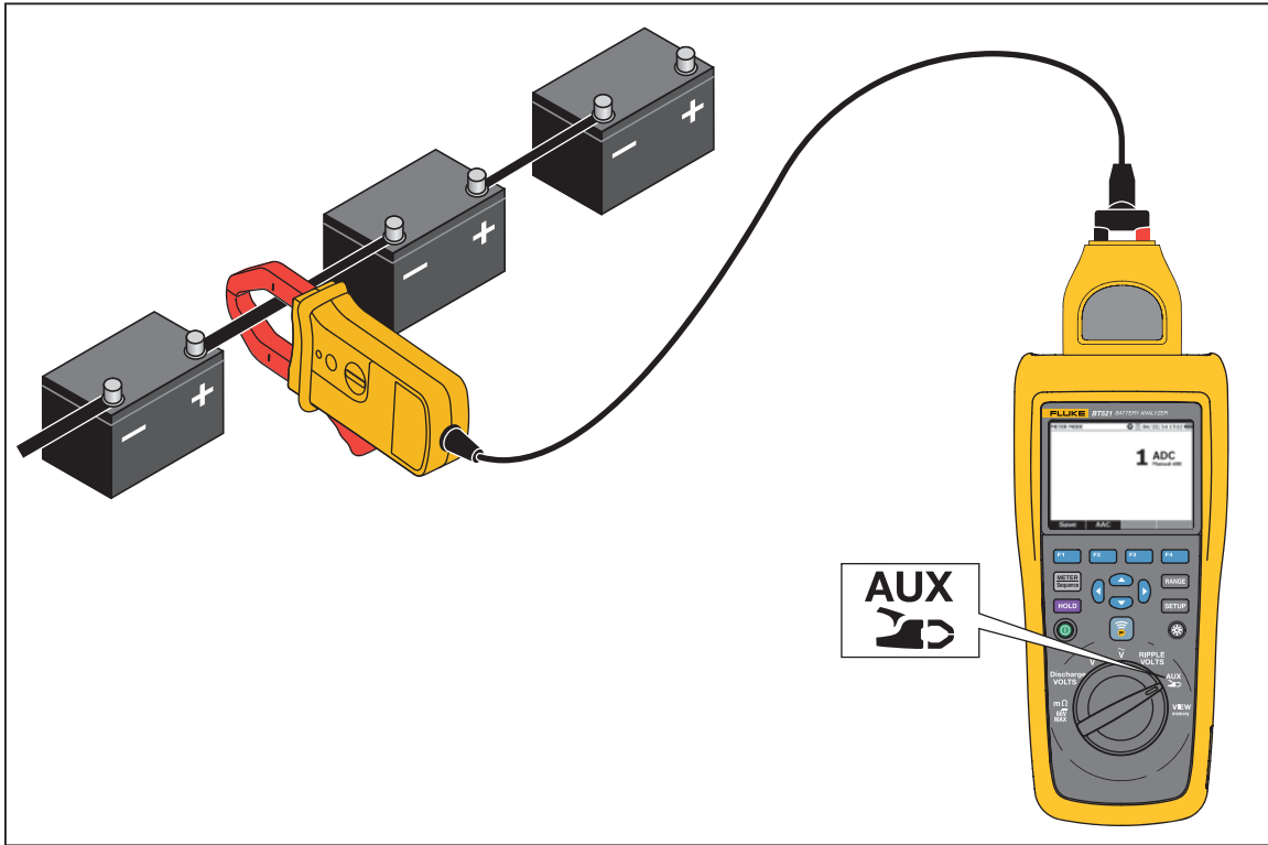
Рис. 3-5. Функция AUX
