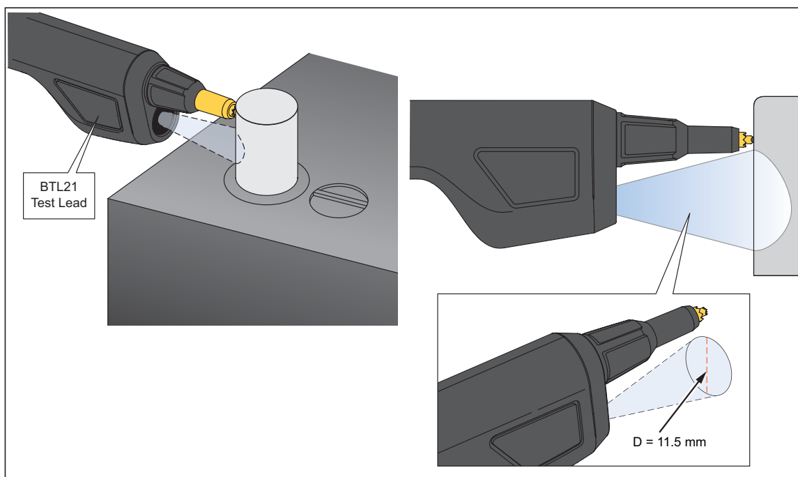
Рис. 4-6. Измерение температуры полюса батареи
