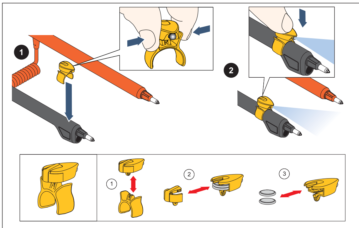
Рис. 4-4. Съемный фонарик
