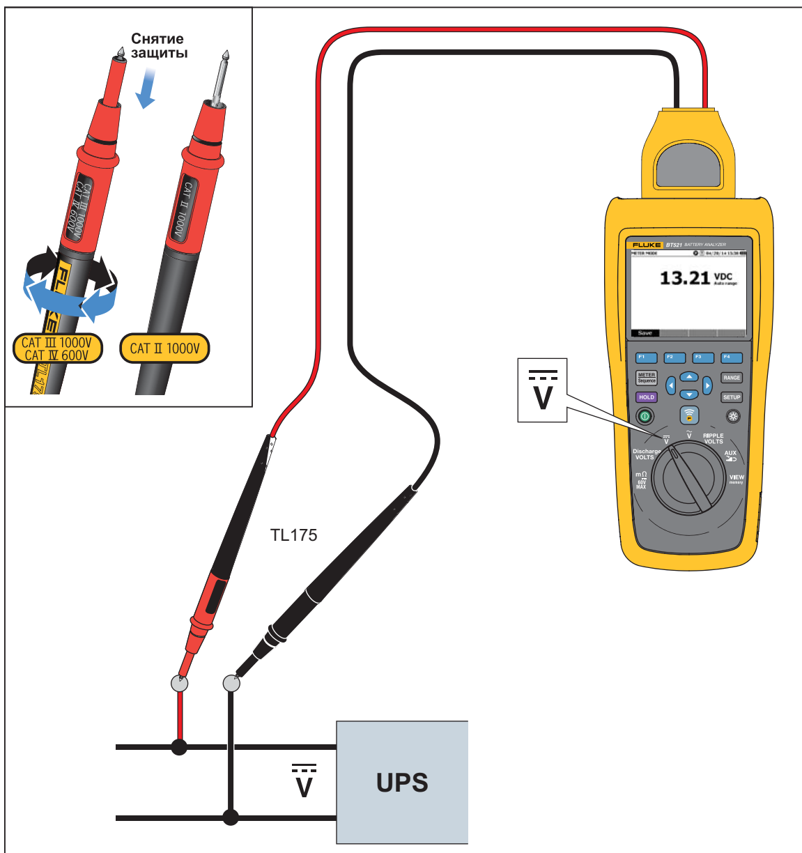
Рис. 3-6. Измерение напряжения постоянного тока с помощью TL175
