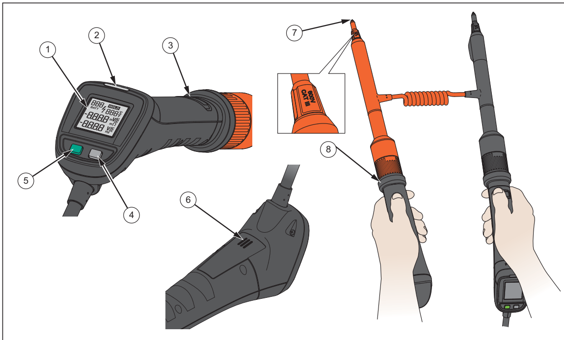
Рис. 4-1. BTL21 Interactive Test Probe
