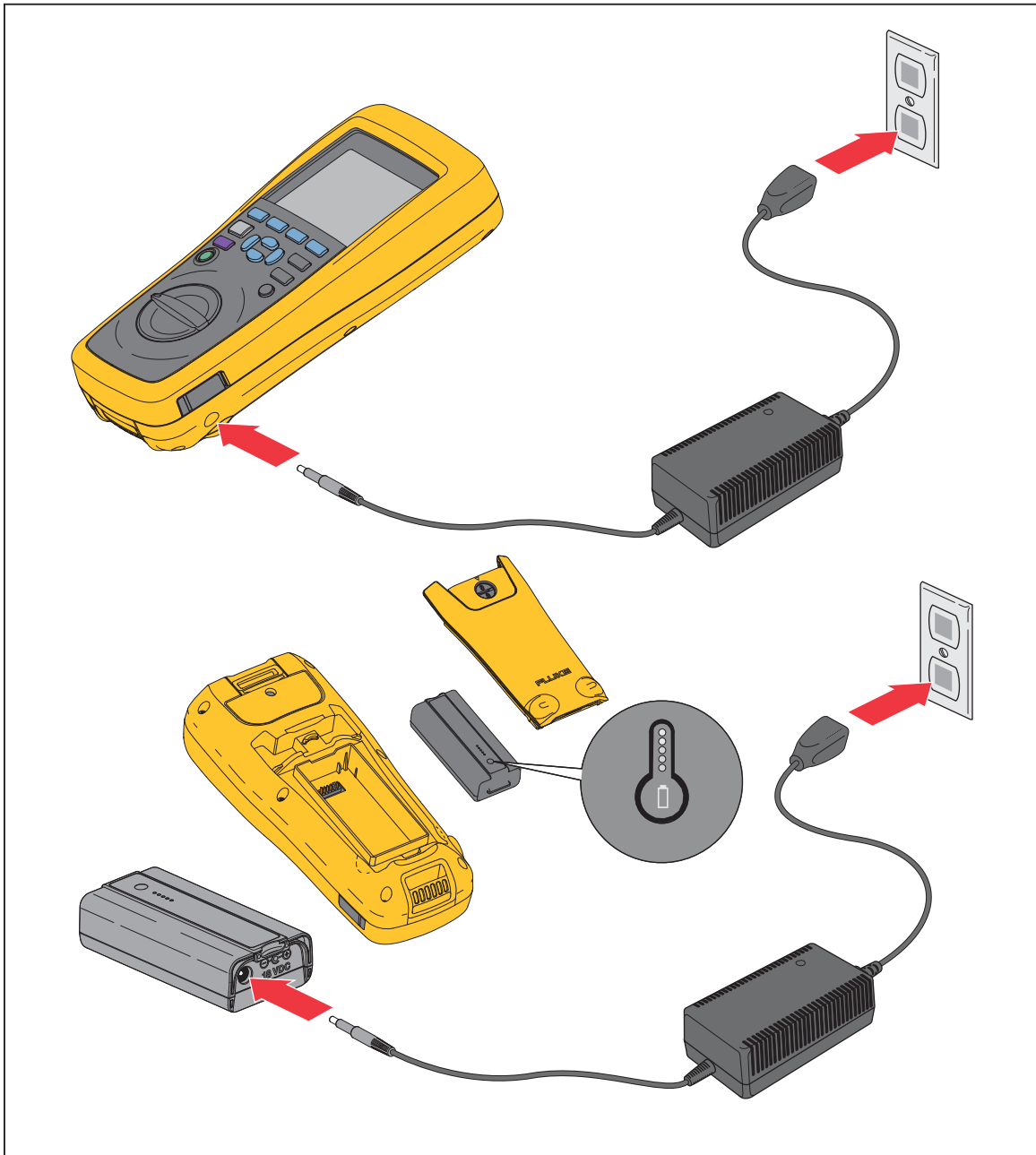
Рис. 6-5. Зарядка батареи
