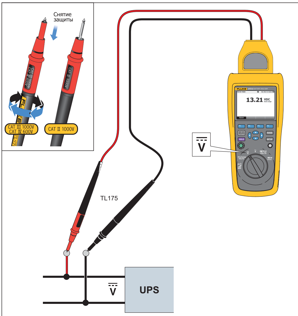
Рис. 3-5. Измерение напряжения постоянного тока с помощью TL175
