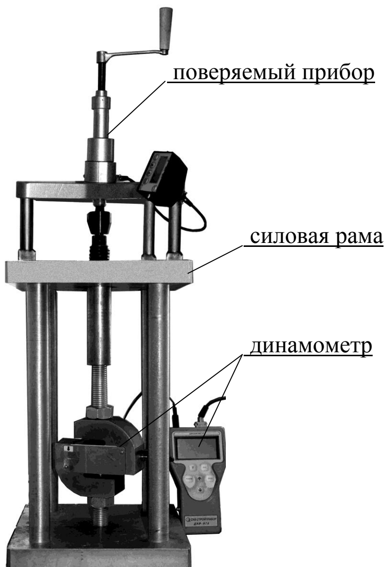
Рисунок 9 – Установка прибора при поверке
