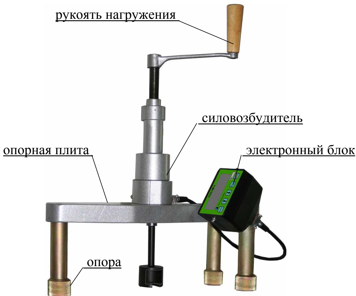
Рисунок 1 - Общий вид прибора ПСО-МГ4К
