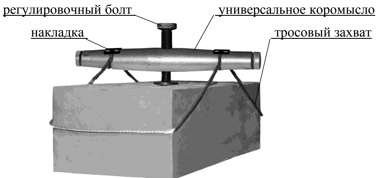
Рисунок 2 – Схема захвата кирпича, подготовленного к испытанию
