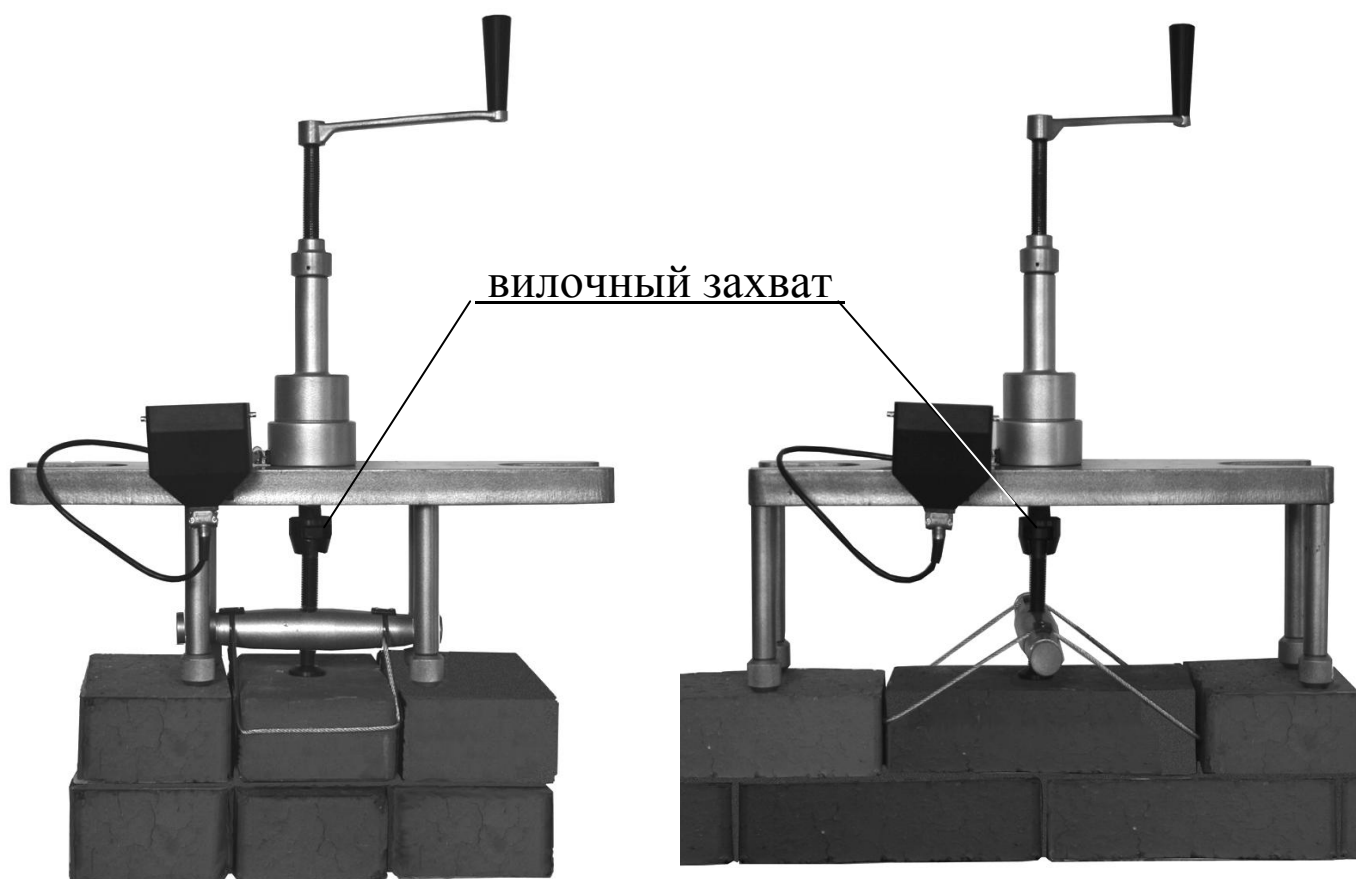
Рисунок 3 – Варианты установки прибора при испытании кирпича
