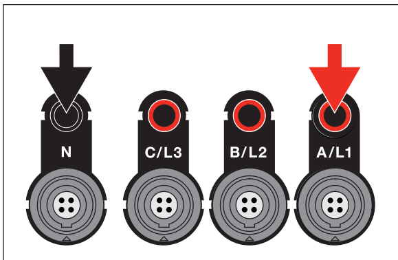
Рисунок 6. Сетевое напряжение с нейтралью
