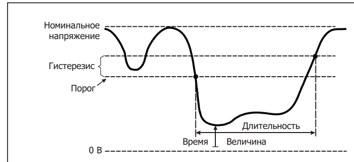
Рисунок 11. Характеристики прерывания напряжения
