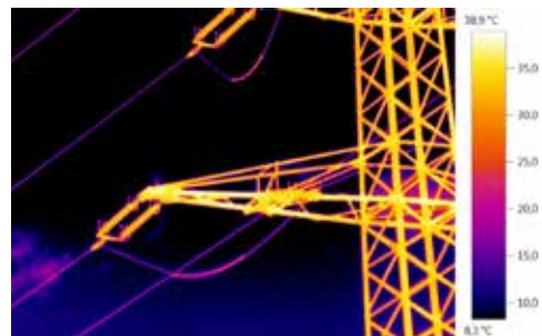
Тепловизионная съемка токового контура на концевой анкерной опоре ЛЭП (расстояние до объекта примерно 120 м)
