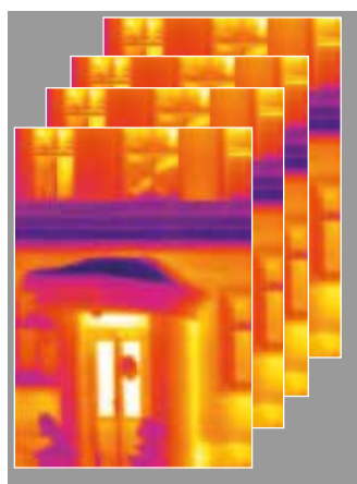
Термограммы
