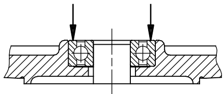
Рис. 13 Подшипник, давление на наружное кольцо
