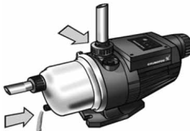
Рис. 12 Опорожнение насоса
