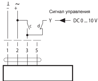
Принудительное управление (схема защиты от замерзания)
