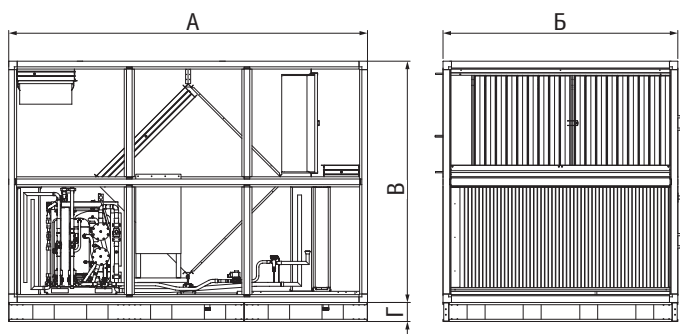
Рекуператор с горизонтальным внутренним клапаном
