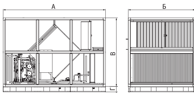
Рекуператор без клапана
