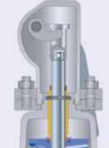
Кольцевой гаситель вибраций H4
