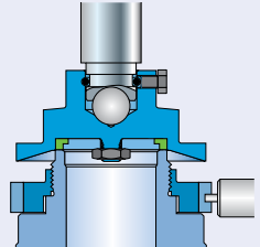
Герметичный колпак H2
