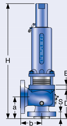
Конструкция с уравновешивающим сильфоном из нержавеющей стали
