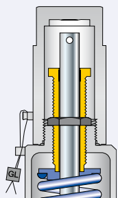
Пневматическое устройство подрыва H8 H8 с одним поршнем
