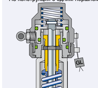
Пневматическое устройство подрыва H8 H8 конструкция с одним поршнем
