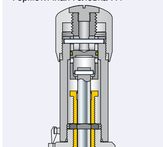
Герметичное устройство подрыва H4 Герметичная головка H4
