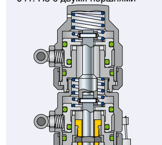
Пневматическое устройство подрыва H8 J41: H8 с двумя поршнями
