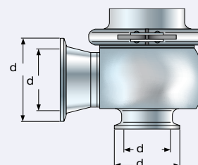
Тип 483 – Диаметр хомутыого соединения
