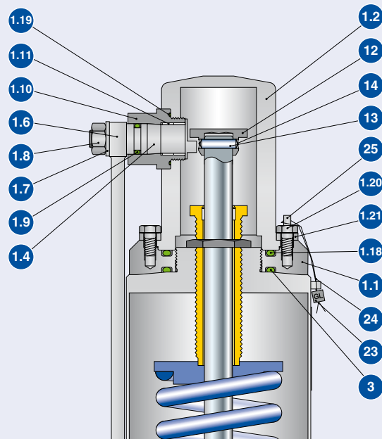
Герметичный рычаг Н4 Размер III
