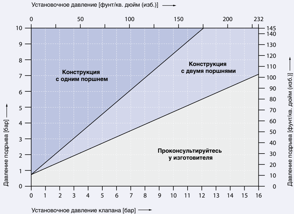
Диаграмма подбора устройства подрыва H8, размер II. d_0 46 мм / 1,811 дюйма
