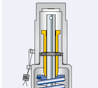
Диск с упл. кольц.
