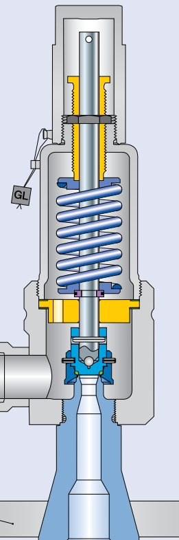
Стандартная конструкция Фланцевое соединение
