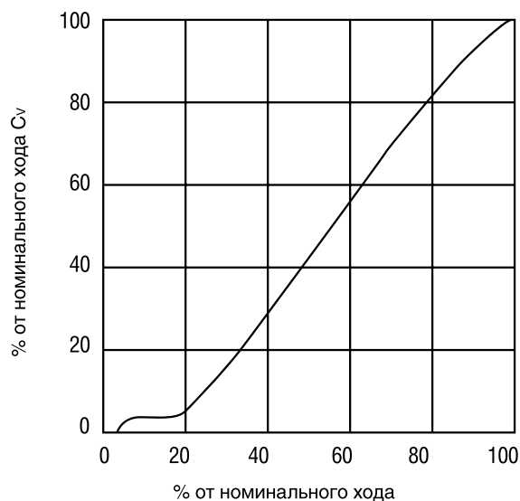
Пропускная способность C_v в зависимости от хода
