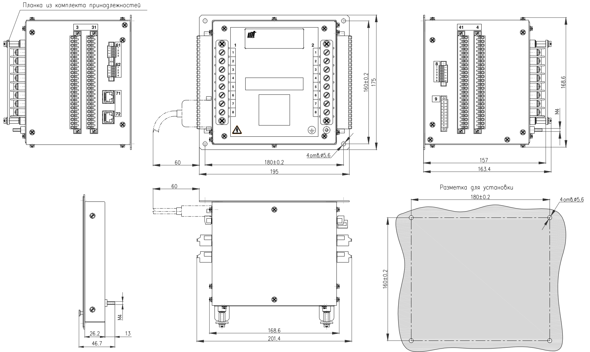
Габаритные размеры пульта 195 x 175 x 46.7 Разметка для установки пульта – в соответствии с рисунком 3а)
