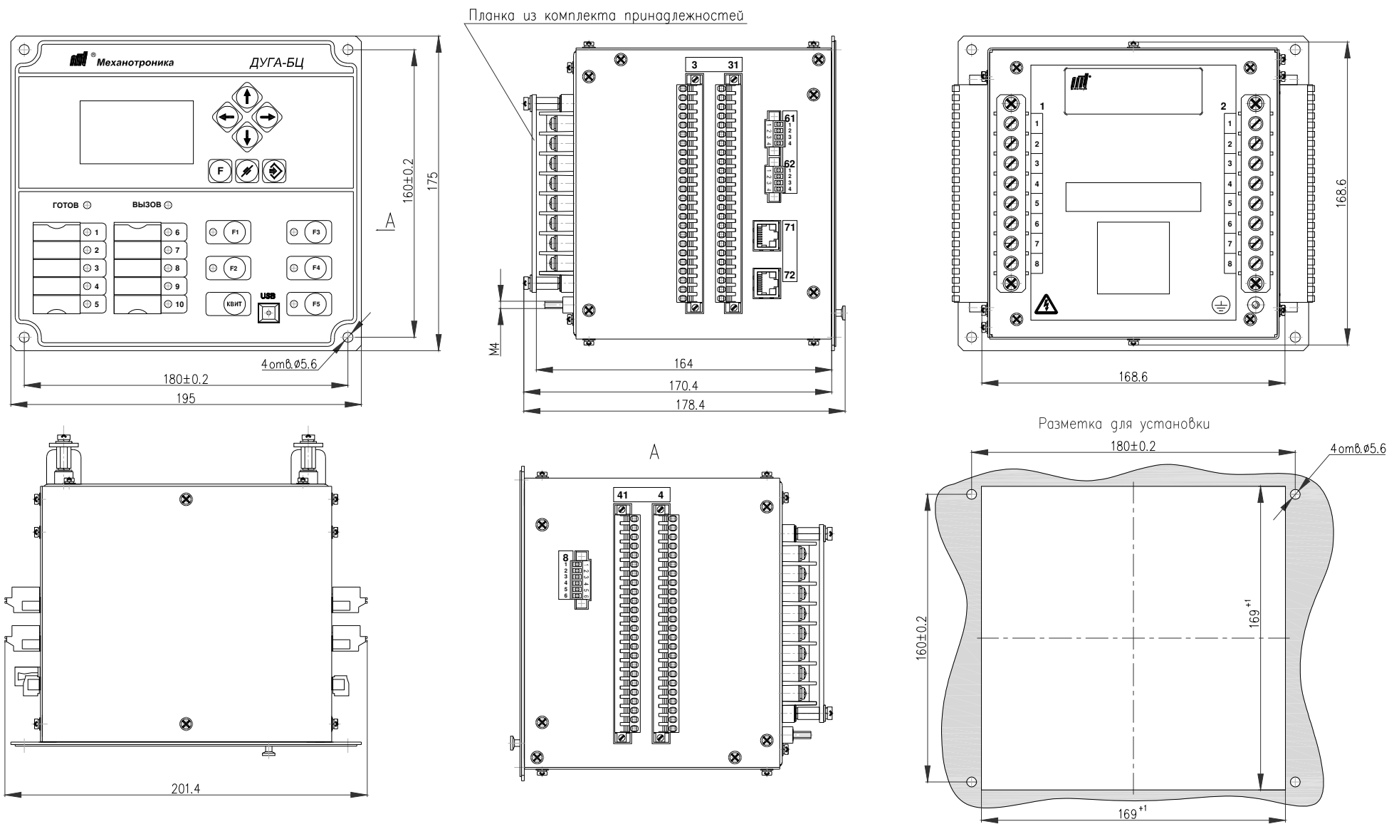
Рисунок 3 (лист 1 из 2) а) - Габаритные и установочные размеры блоков ДИВГ.421452.007, ДИВГ.421452.107
