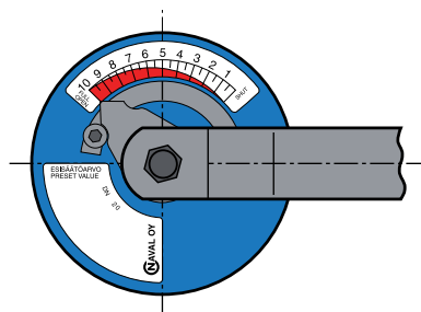
ШКАЛА РЕГУЛИРОВКИ (КРАНЫ С РУЧКОЙ) DN15-32
