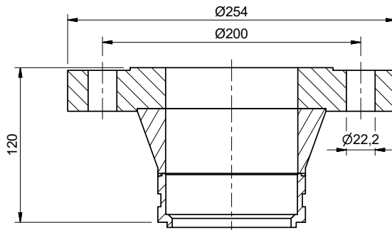
IN100 (4" - 300 Lb)
