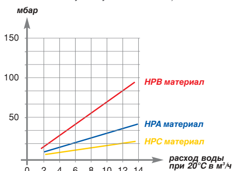
Пропускная способность / Δ P схемы для высокоэффективного мешочного фильтра HP – размер 10
