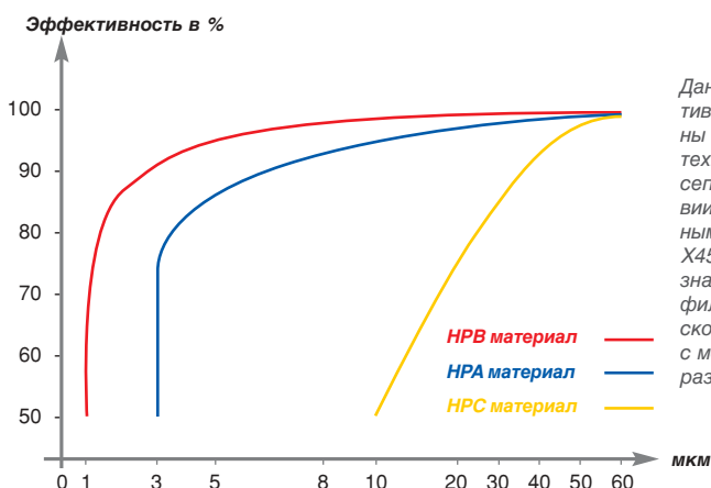
Эффективность высокопроизводительных мешочных фильтров HP
