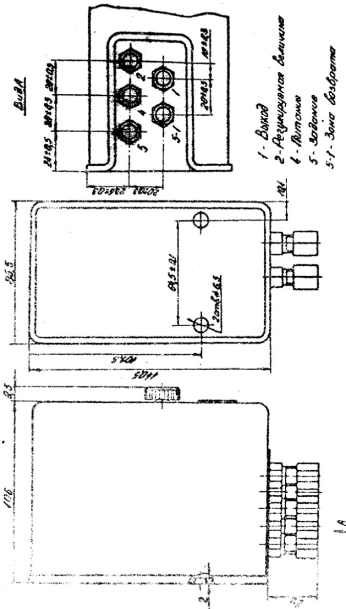
Рис. 3. Габаритные и установочные размеры регулятора
