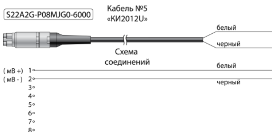
Рисунок А.9 – Соединительный кабель «КИ2012U» для связи ИКСУ с первичными преобразователями или устройствами при работе в режиме измерений напряжения постоянного тока, а также воспроизведения сигналов напряжения постоянного тока
