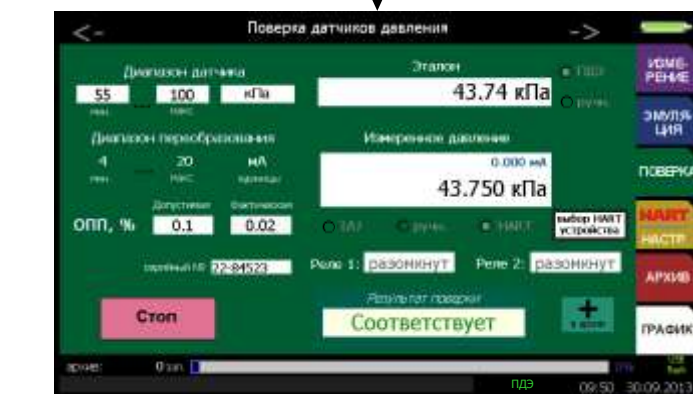
Рисунок 2.87 – Поверка датчиков давления
