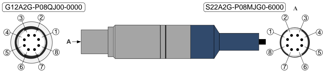
Рисунок А.1 – Разъемы для измерения сигналов от ТП, мА, мВ, В; ТС, Ом и воспроизведения сигналов от ТП, мА, мВ, В
