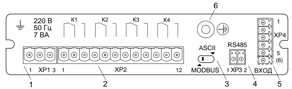
Рисунок 2.4 – Задняя панель ИРТ 5940/M1
