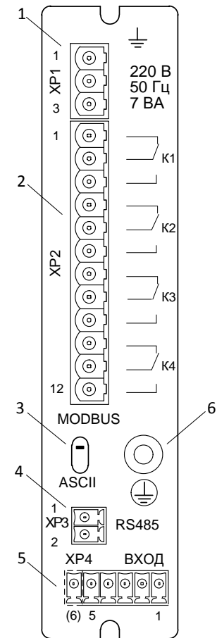
Рисунок 2.5 – Задняя панель ИРТ 5940/M2
